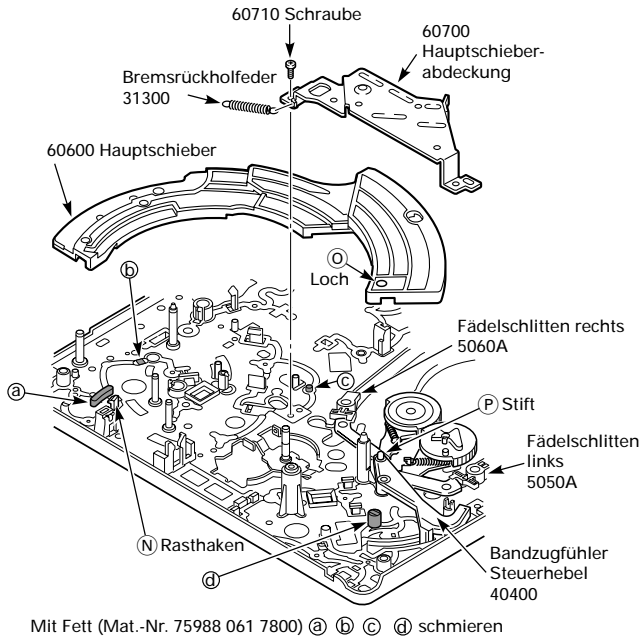
Mit Fett (Mat.-Nr. 75988 061 7800) a) b) c) d) schmieren
